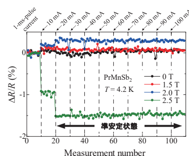
電流パルスで磁気状態が変化し、抵抗値が切り替わる様子
