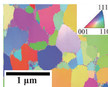
電子の回折現象を用いて可視化された半導体多結晶薄膜の結晶構造分布
