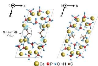
リン酸八カルシウム: \text{H}_2\text{O} の有無が原子・電子構造に与える影響
