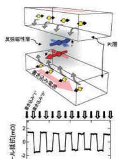
反強磁性体磁気メモリの実証
